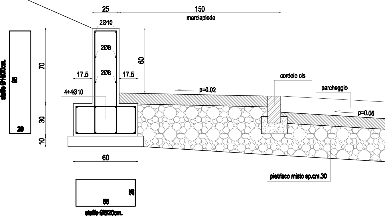
PARTICOLARE COSTRUTTIVO scala 1:20
