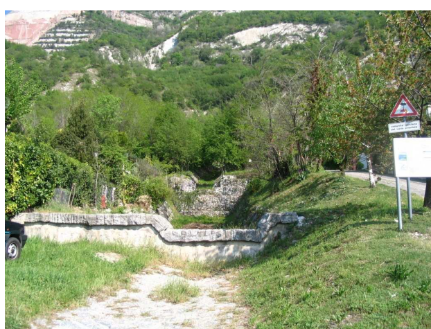
Tratto apicale della Valle Cepelline a monte del guado di Via Manzoni. In primo piano briglia in cls e pietrame. In secondo piano briglia in gabbionate.
